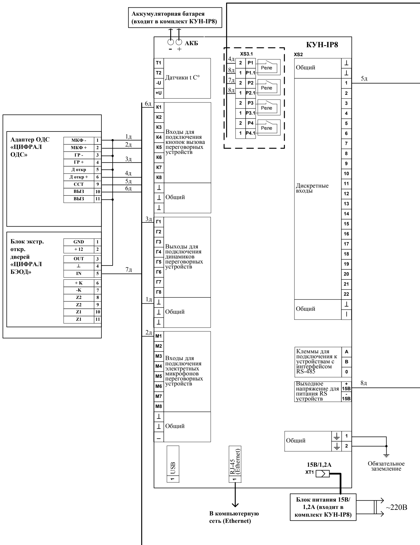
Рис. Б 4.2.2-2 Схема подключения КУН-IP8 с адаптером ОДС домофона «ЦИФРАЛ»
