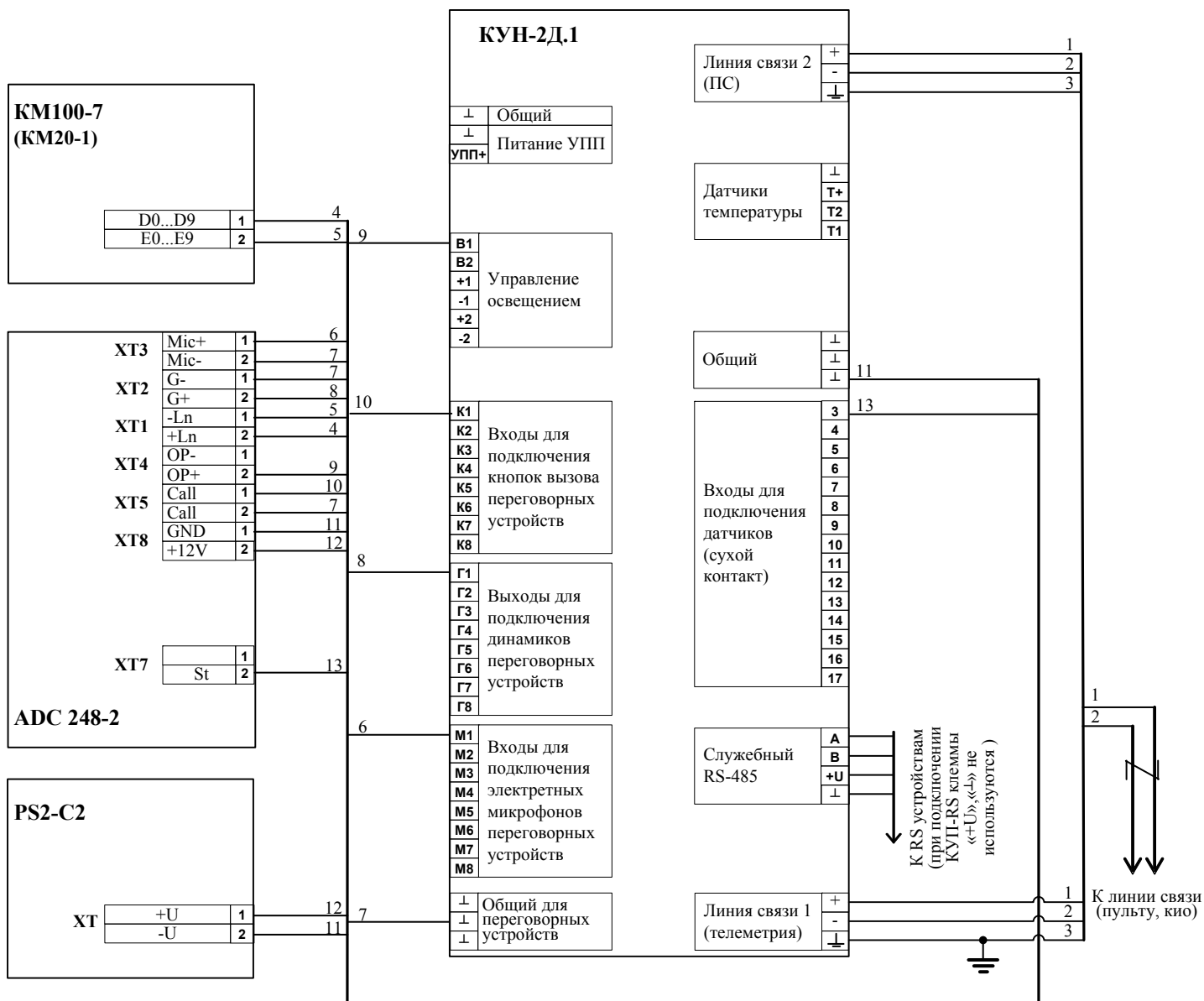
Рис. Б 4.2.3-2 Схема подключения КУН-2Д.1 и адаптера ADC 248-2 домофона «Элтис»
