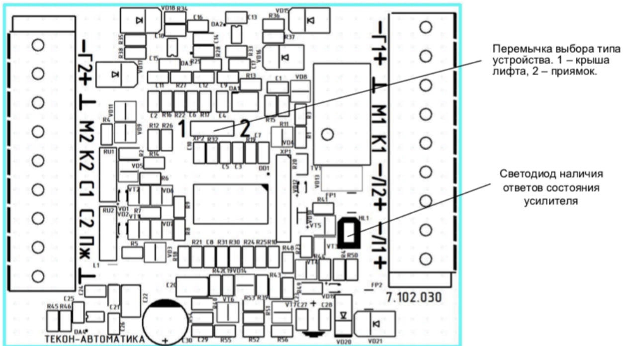
Рисунок 1 – Схема расположения светодиодов и перемычек на УПУ-М
