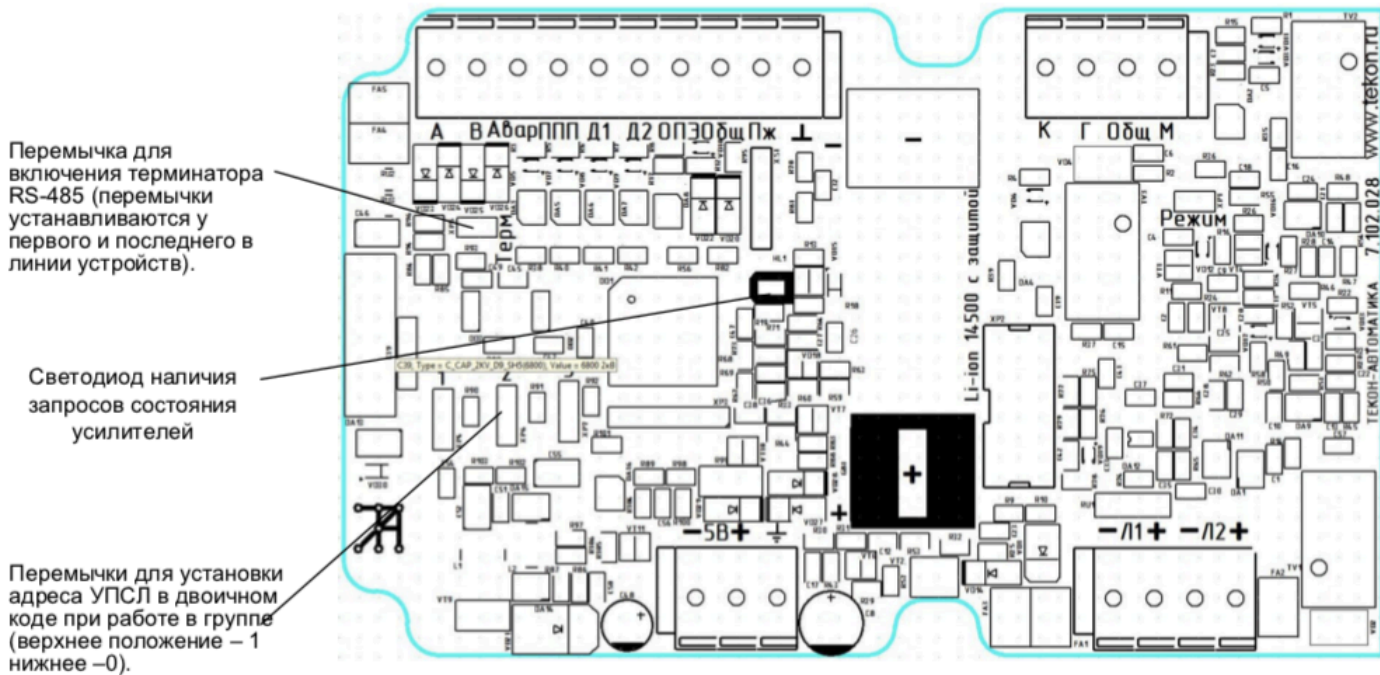
Рисунок 2 – Схема расположения светодиодов и перемычек на ПУ-М
