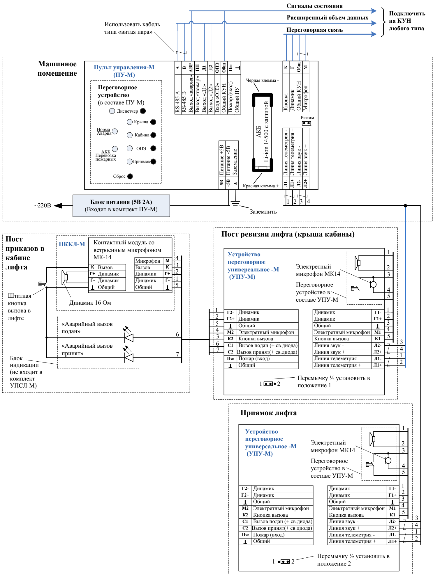
Рис. Б 2.20.3 Устройство переговорной связи лифта - М исполнение 1 (УПСЛ-М исп.1). В комплект входит ПУ-М – 1 шт., УПУ-М – 2 шт., ПККЛ-М – 1 шт. Основные функции: ремонтная связь лифта, связь с помещением для обслуживающего персонала.
