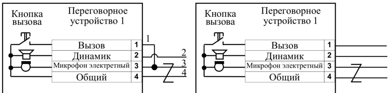
Рис.1. 3-х.проводная схема
