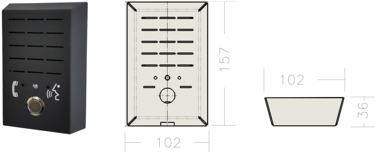
Рис.1. Переговорное устройство в антивандальном исполнении (ПГУ схема 14) – накладной монтаж
