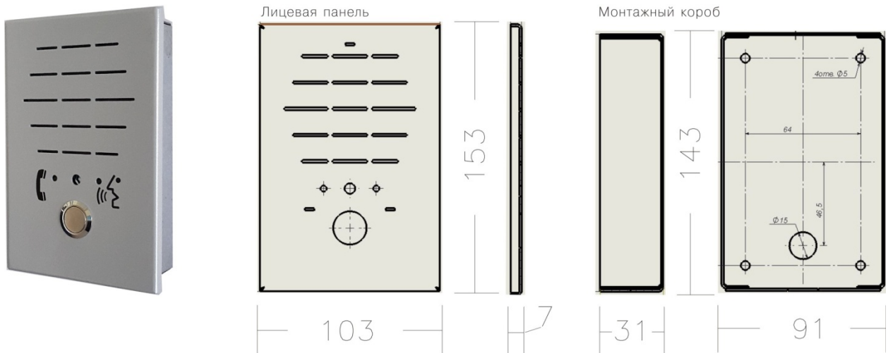
Рис.2. Переговорное устройство в антивандальном исполнении 2 (ПГУ-2) – врезной монтаж
