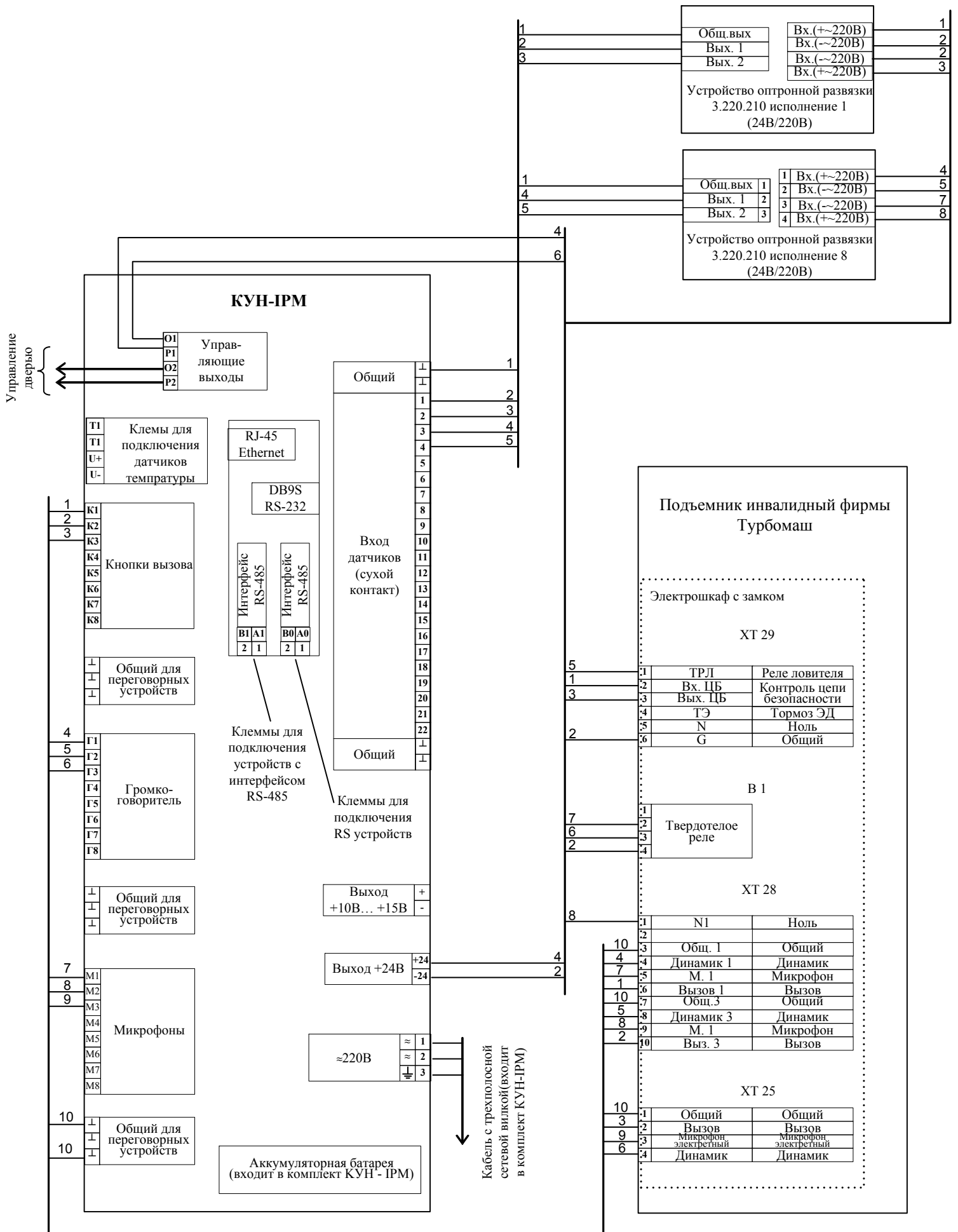
Рис. Б 4.3.2 Схема подключения КУН-IPM к одному подъемнику ПВИ-220 фирмы Турбомаш.
