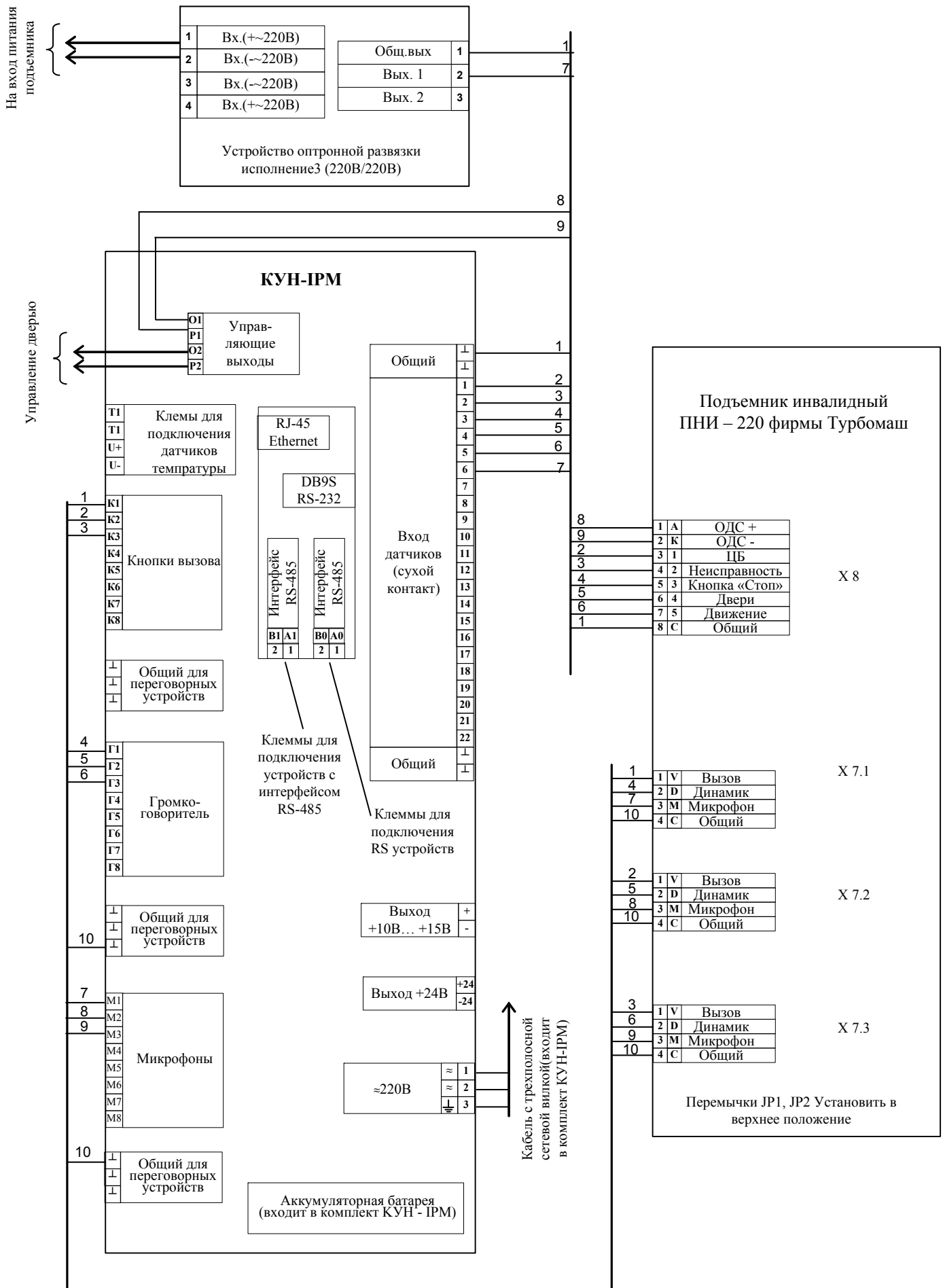
Рис. Б 4.3.3 Схема подключения КУН-IPM к одному подъемнику ПНИ-220 фирмы Турбомаш.
