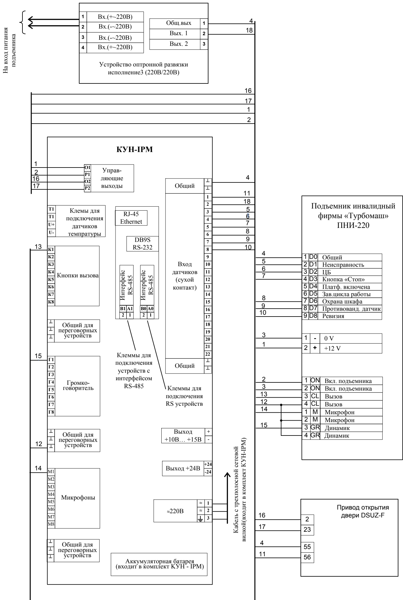
Рис. Б 4.3.7 Схема подключения КУН-IPM к одному подъемнику ПНИ-220 фирмы Турбомаш и к приводу открытия двери DSUZ-F.
