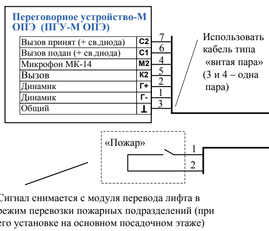
Рис. Б 2.20.4 Устройство переговорной связи лифта - М исполнение 2 (УПСЛ-М исп.2). В комплект входит ПУ-М – 1 шт., УПУ-М – 2 шт., ПККЛ-М – 1 шт., ПГУ-М ОПЭ – 1 шт.). Основные функции: связь лифта для пожарных, ремонтная связь лифта, связь с помещением для обслуживающего персонала.
