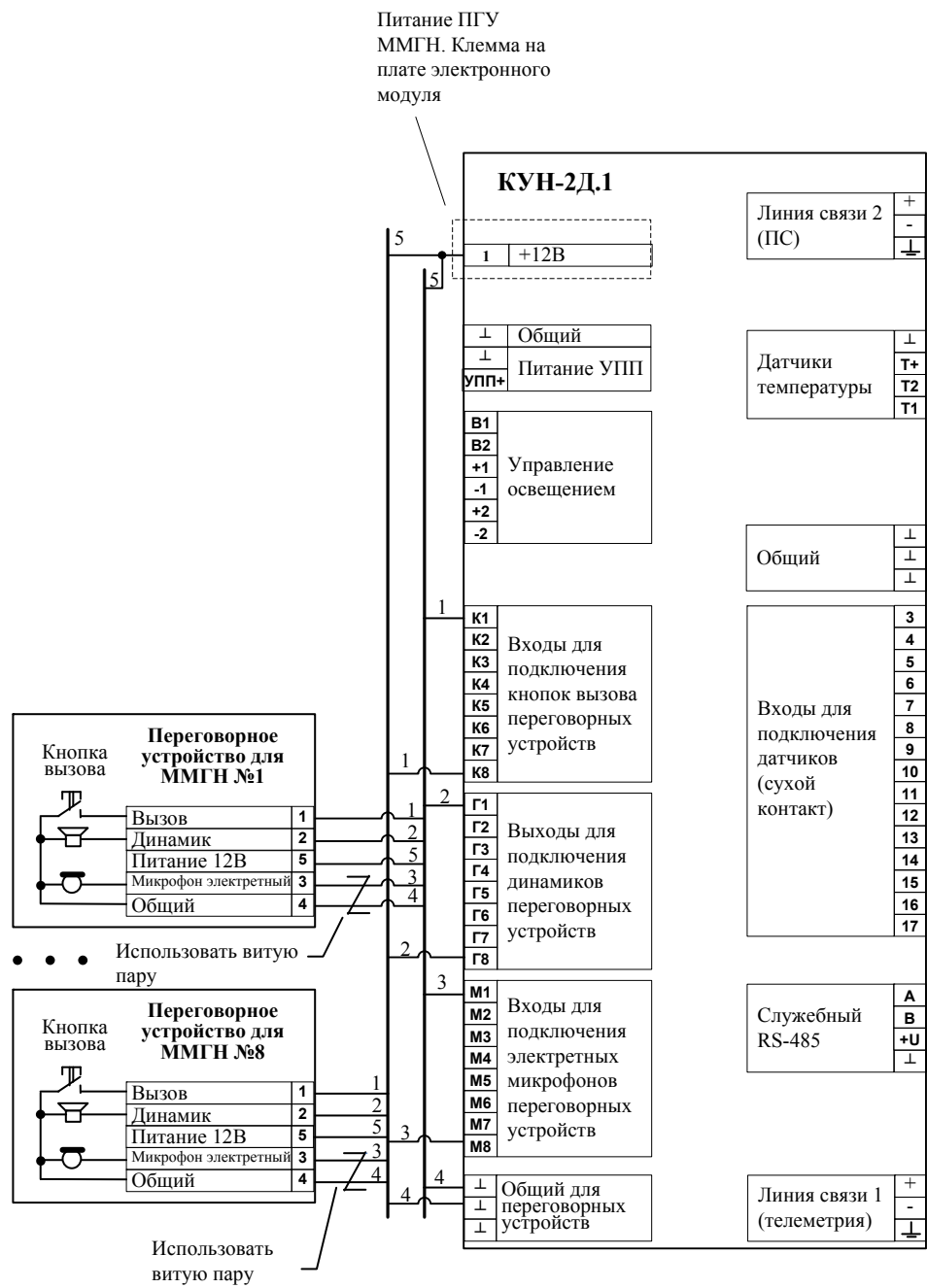
Рис. Б.2.21.1 Схема подключения переговорного устройства в антивандальном исполнении для маломобильных групп населения (ПГУ ММГН) к КУН-2Д.1. Подключение ПГУ ММГН к КУН-IP8, КУН-IP4, КУН-2ДМ осуществляется аналогично. В КУН-IP4 ПГУ ММГН на 4-й. канал ПГС не подключать.
