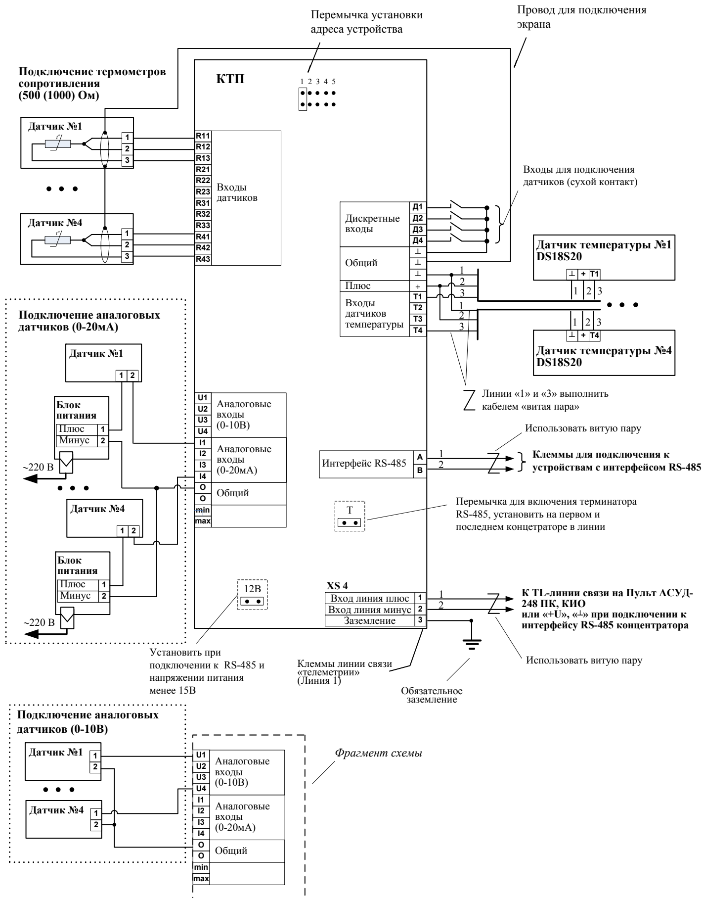
Рис. Б 2.8.1-2 Схема подключения концентратора теплового пункта (КТП) (вариант 1). Подключение КТП к аналоговым датчикам (0-20мА, 0-10В), термометрам с сопротивлением 500 (1000) Ом и цифровым датчикам температуры.
