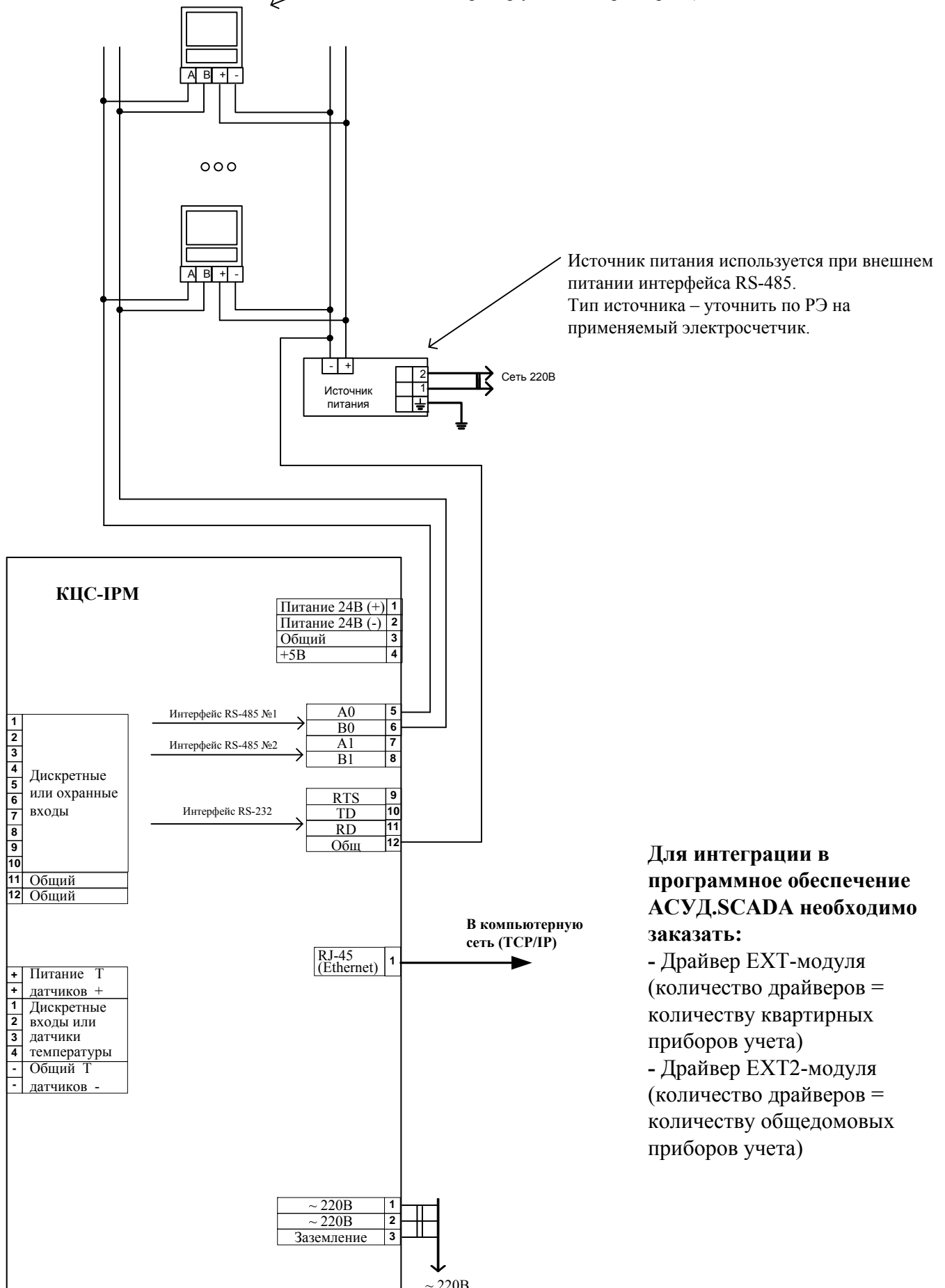
Рис. Б 4.4.1-3 Схема подключения концентратора цифровых сигналов ИРМ (КЦС-ИРМ) и приборов учета электроэнергии по интерфейсу RS-485. Питание интерфейса RS-485 осуществляется от внешнего или встроенного в электросчетчик источника питания.
